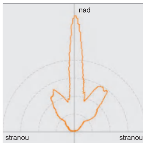
Graf světelného toku LED majáku 230
